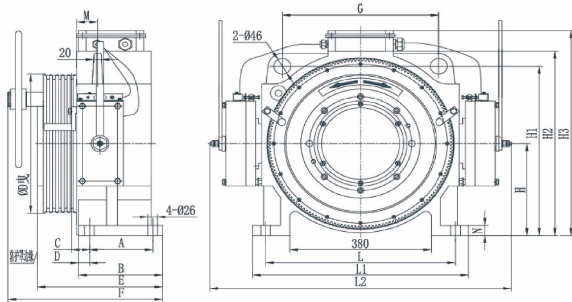
外观尺寸图 | Outline drawing
